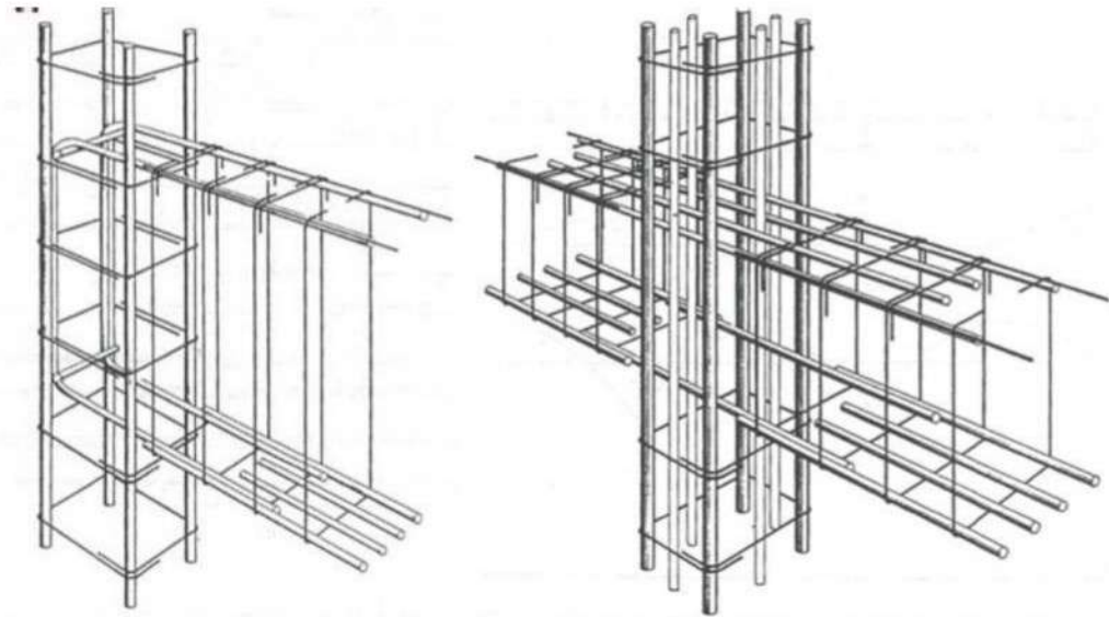
รูปที่ 89 ตัวอย่างการวางเหล็กคานผ่านเสา
