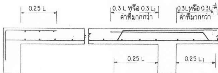
รูปที่ 90 ระยะตัดคอกำ และการจัดเหล็กพิเศษตามมาตรฐาน ACI พื้นคอนกรีตเสริมเหล็กที่มีความหนาต่างระดับกัน การดุ้งเหล็กเอียง
